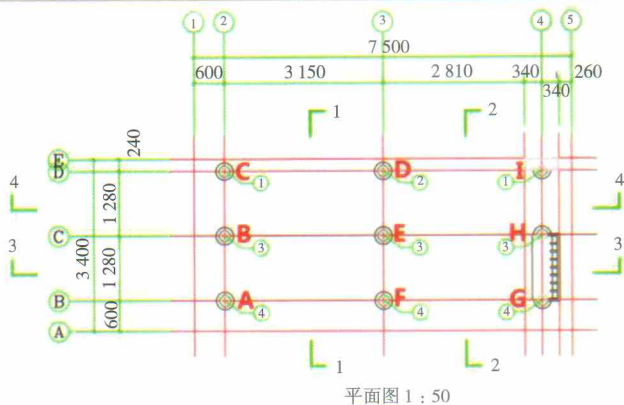
图4 木结构试验亭平面图(图片来源:陈琳策划,孙启祥绘)
