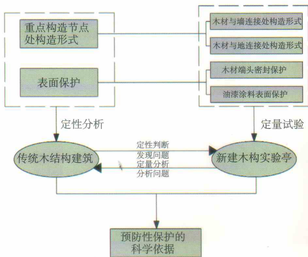
图3 传统木结构建筑预防性保护的定性研究与定量研究过程图 (图片来源:作者自绘)
